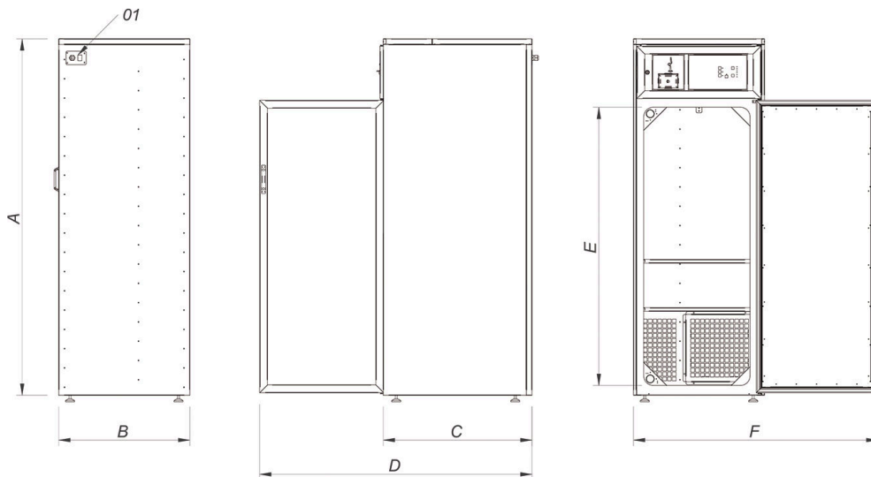
01. Conexión eléctrica
