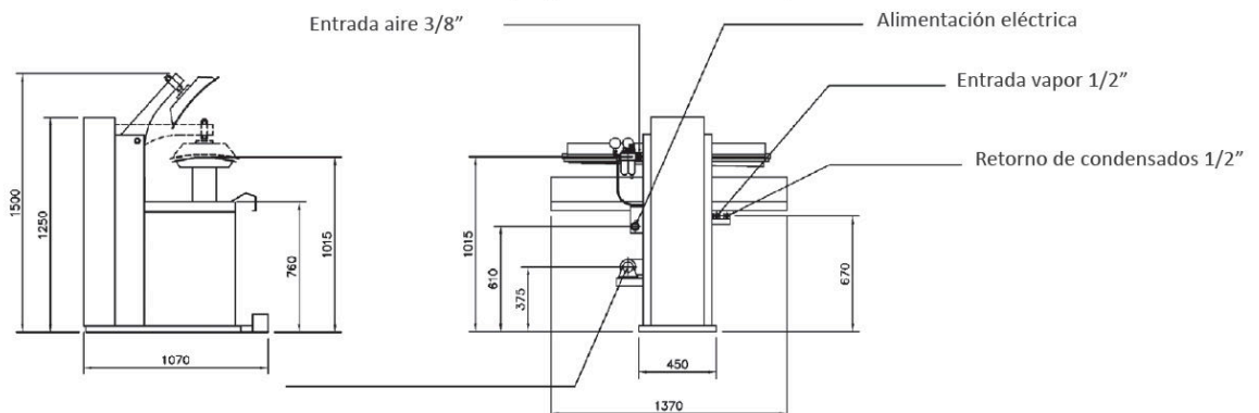
UB / CPB CENTRALIZADA (SIN CALDERA)
